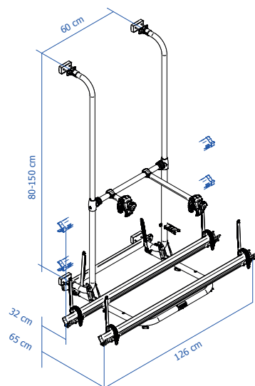
Thule Sport G2 - Standard
