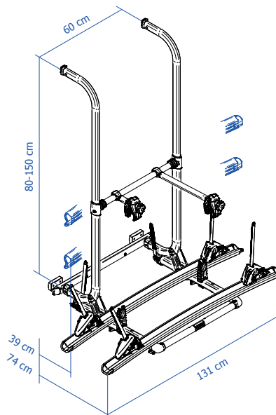
Thule Elite G2 - Hymer Hooks
